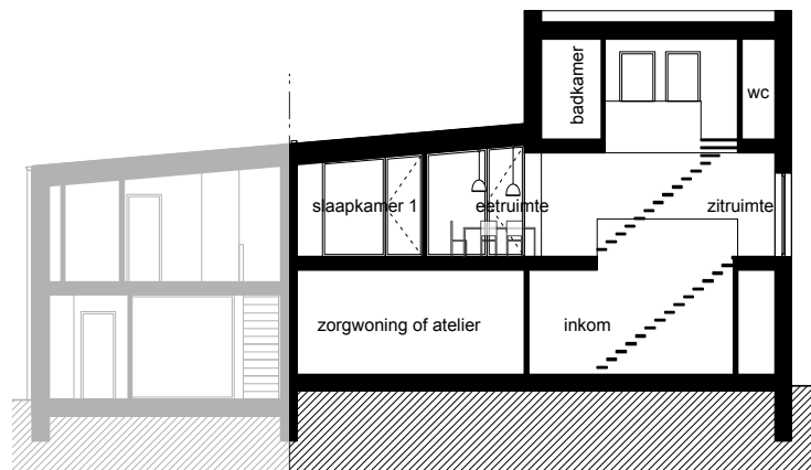
SNEDE AA' 1/200
