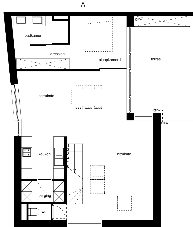
NIVO +1 A'
