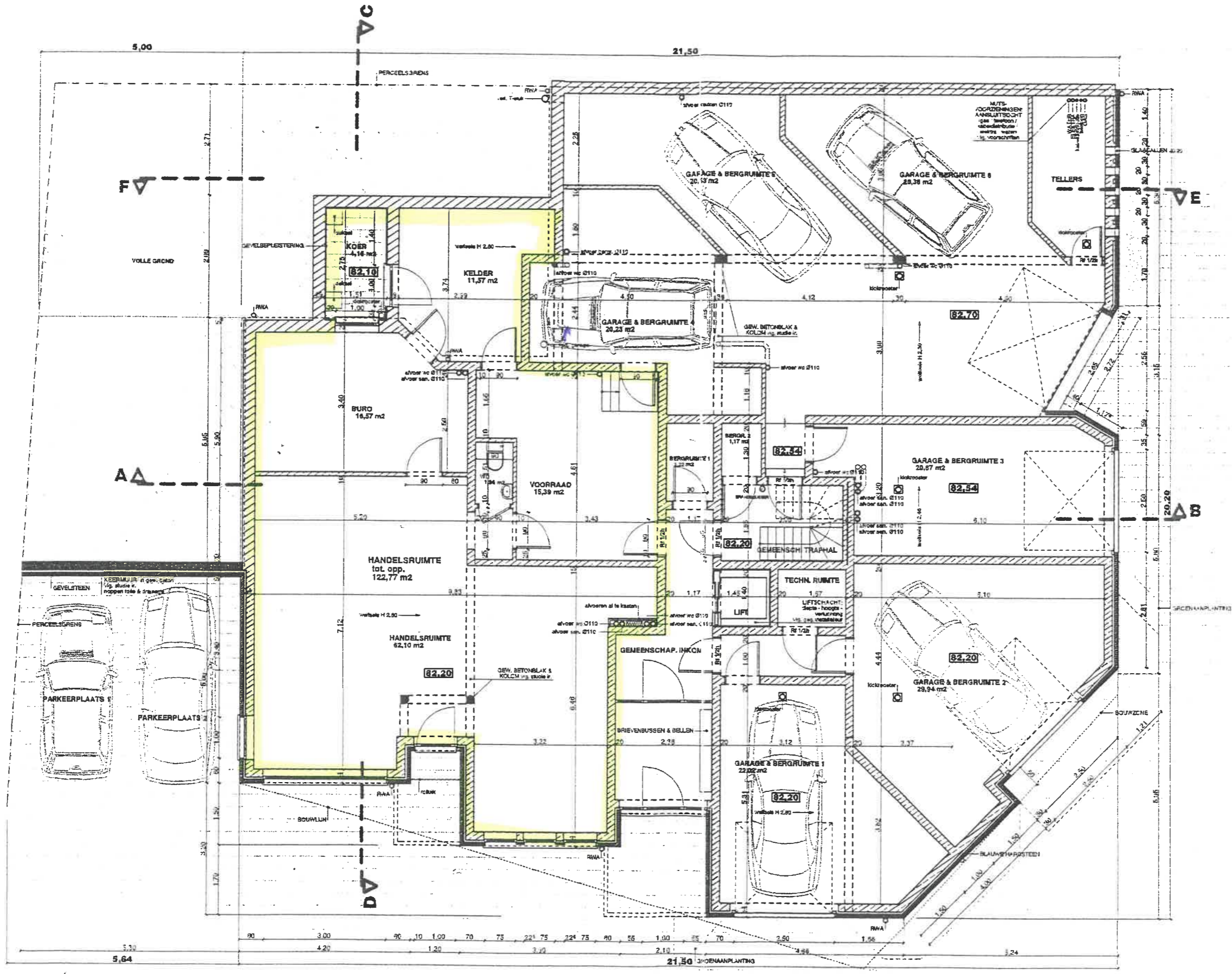
GELIJKVLOERS schaal 1/50
