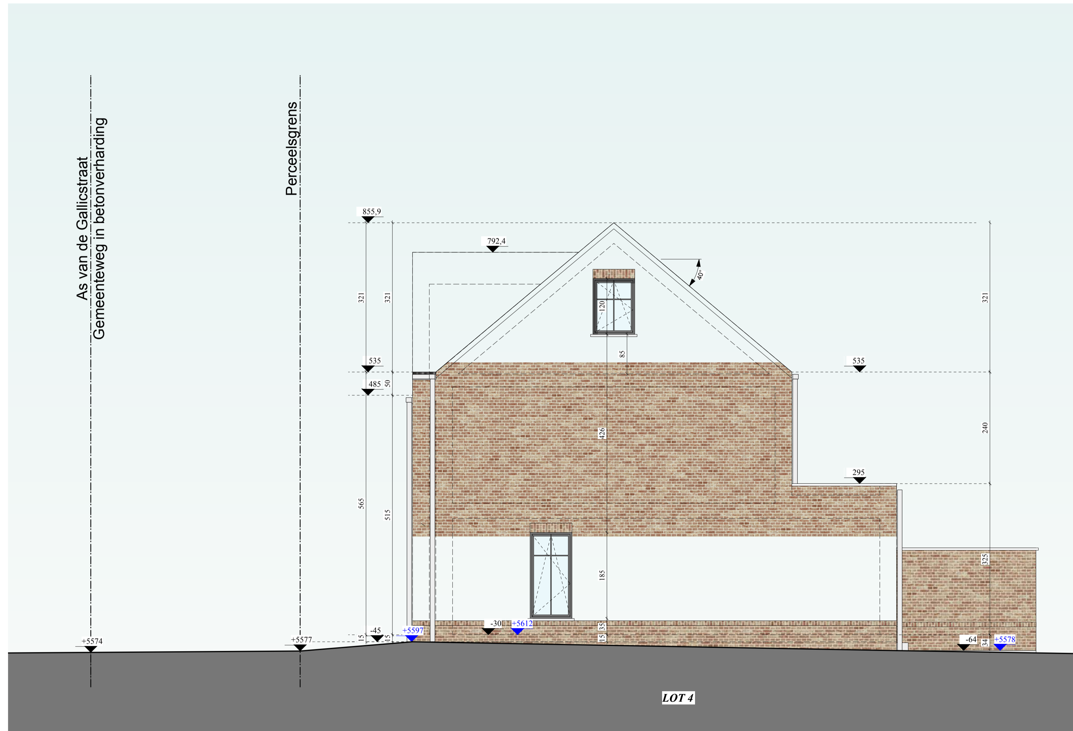
LOT 4 - RECHTERZIJGEVEL
