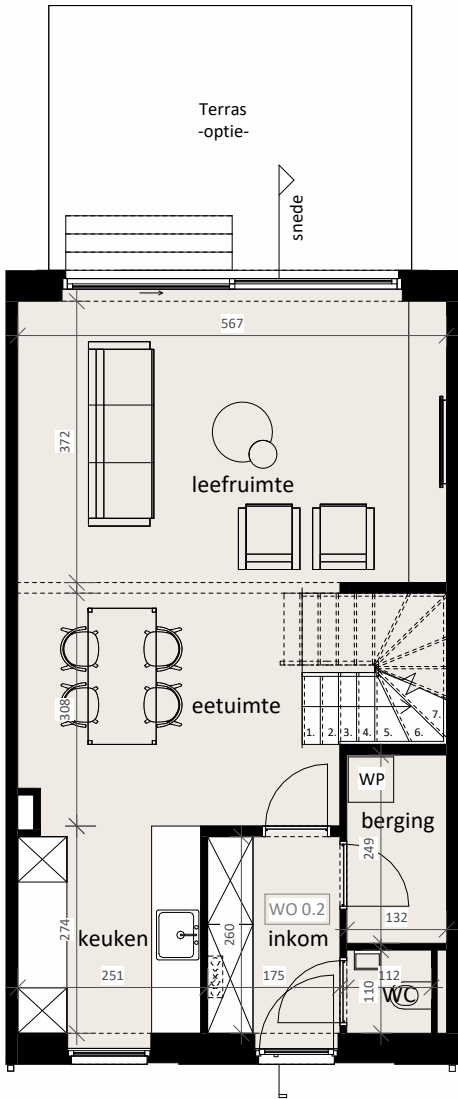
GELIJKVLOERS 1:100
