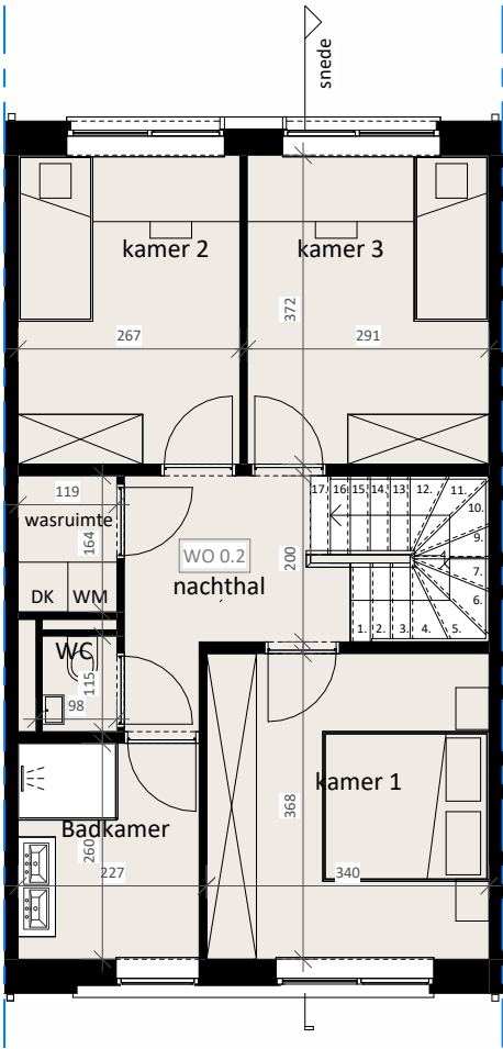
EERSTE VERDIEPING 1:100
