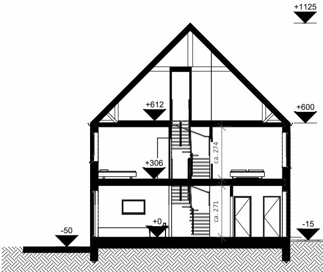
SNEDE 1:200
