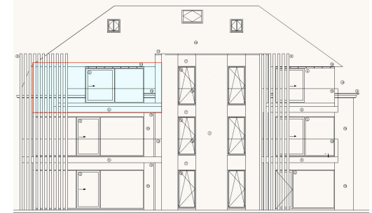
ACHTERGEVEL (NW)
