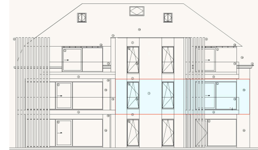
ACHTERGEVEL (NW)
