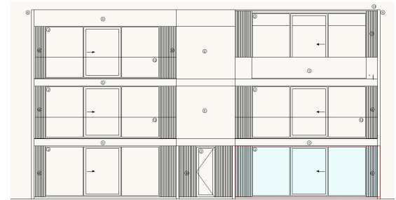
VOORGEVEL (ZW)
