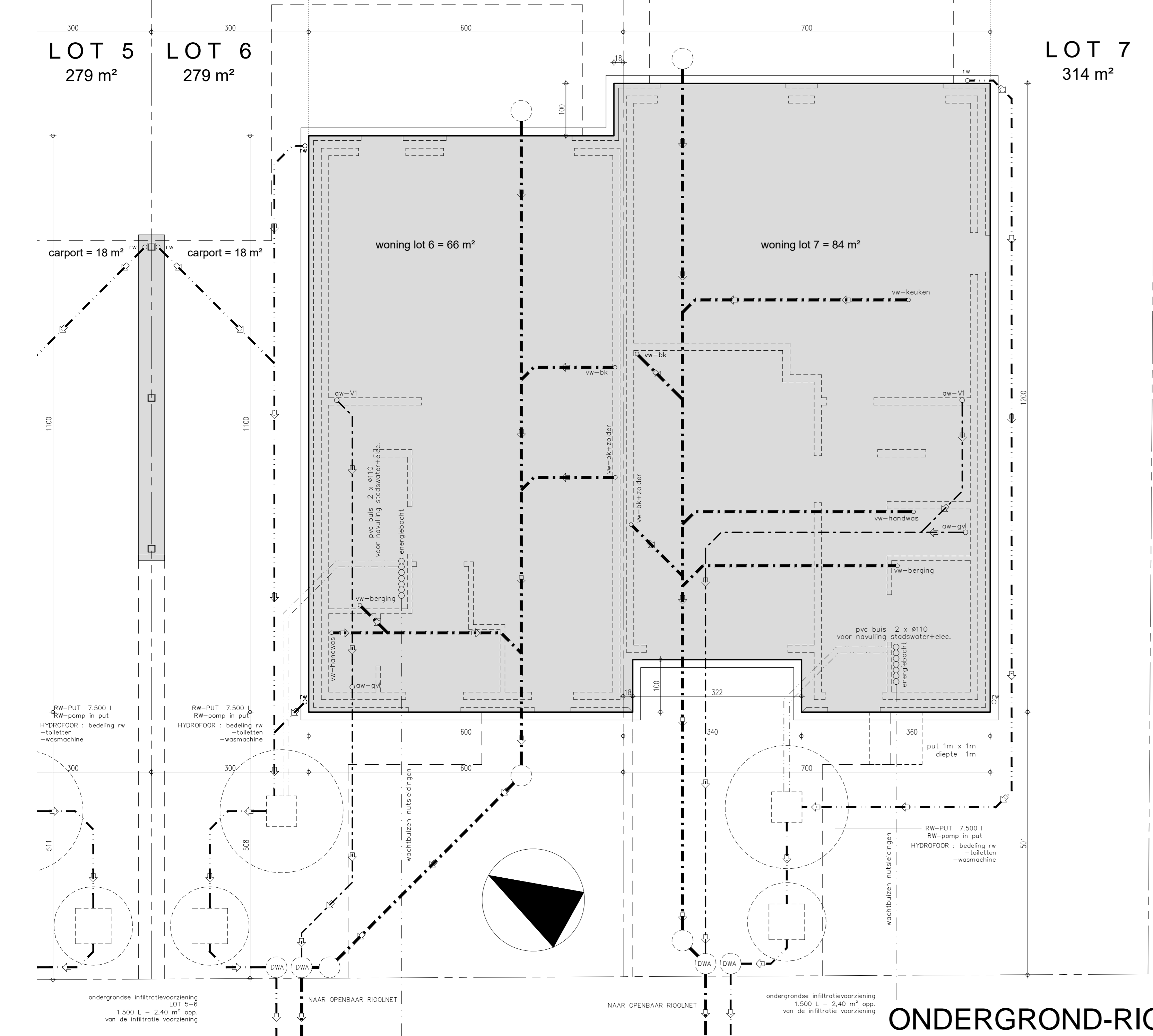
ONDERGROND-RIOLERING 1/50
